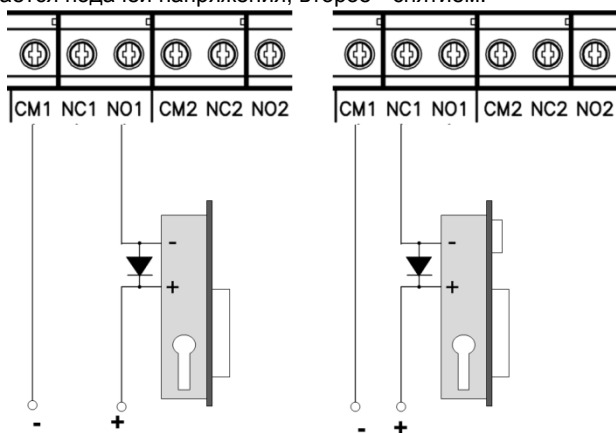
Рис.13. Подключение замков
