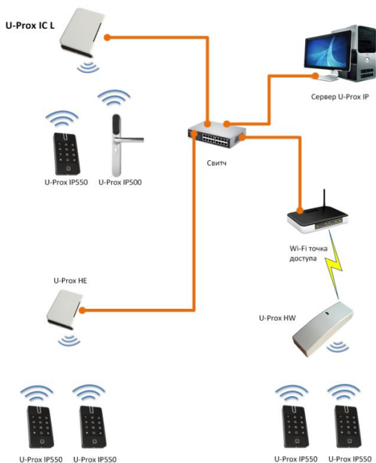
Рис 3. Пример локальной сети смешанного типа (Ethernet и Wi-Fi)
