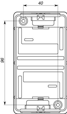
Рис 8. Задняя пластина
