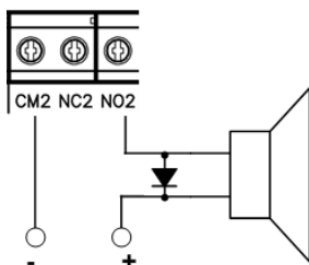
Рис. 14. Подключение электрозвонков
