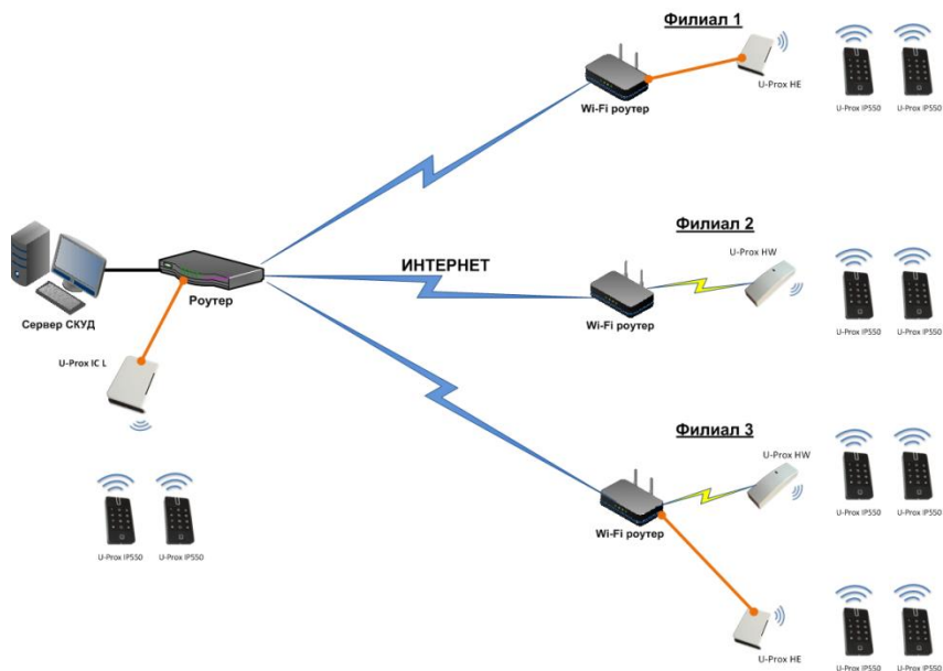
Рис 4. Пример распределенной сети
