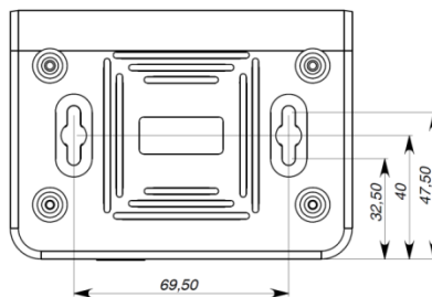
Рис 8б. Разметка крепежных отверстий, модификация 2
