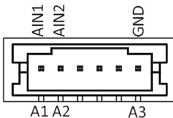
Рисунок 4-3 Разъемы DS-KH6310-WL/DS-KH6210-L
