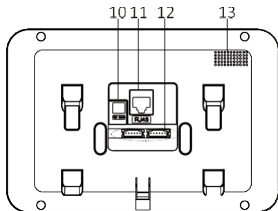
Рисунок 2-4 Задняя панель
