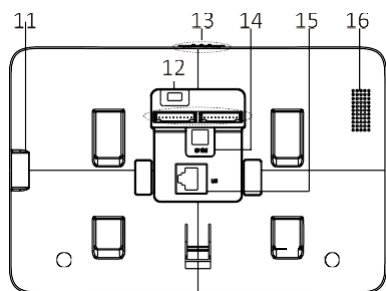
Рисунок 2-2 Задняя панель
