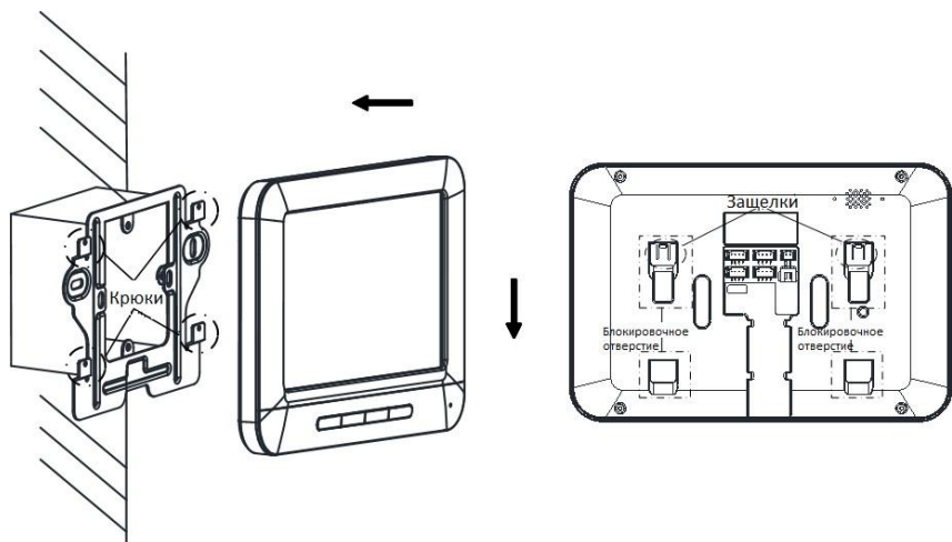
Рисунок 5-3 Крепление видеодомофона
