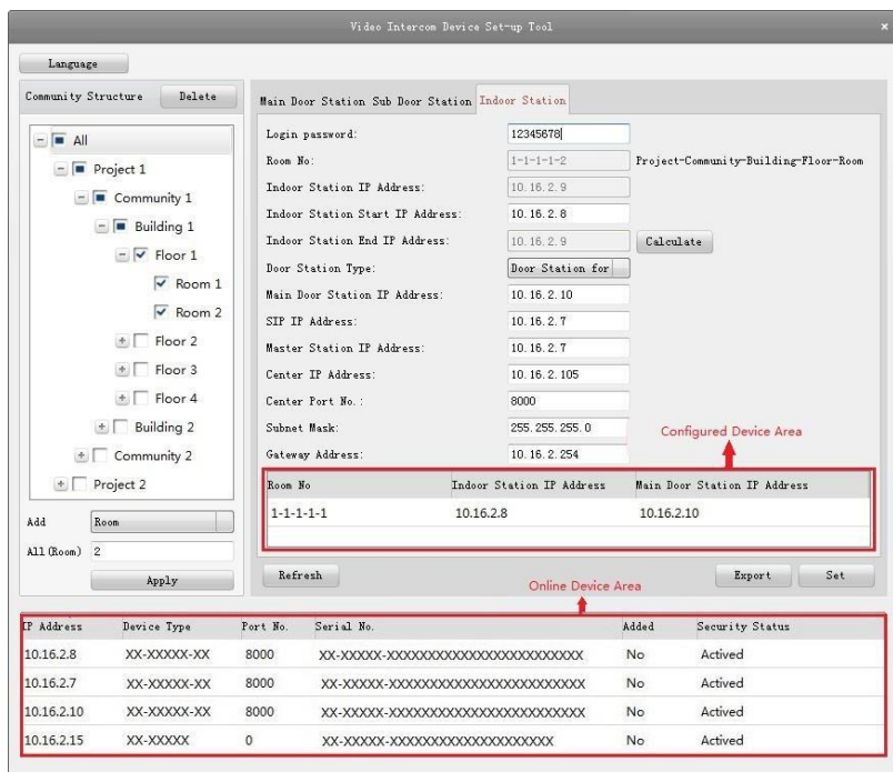
Рисунок 8-37 Настройка домофона
