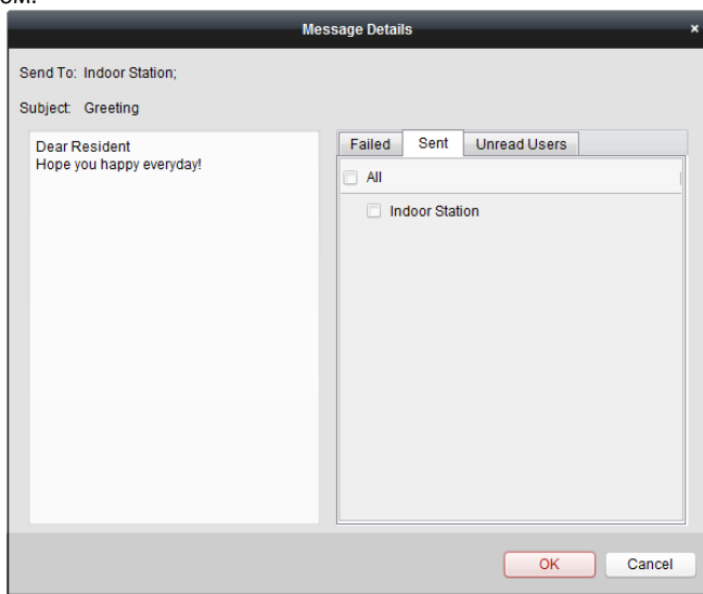
Рисунок 9-42 Детали сообщения
