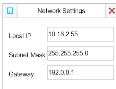
Рисунок 7-22 Настройка сети
