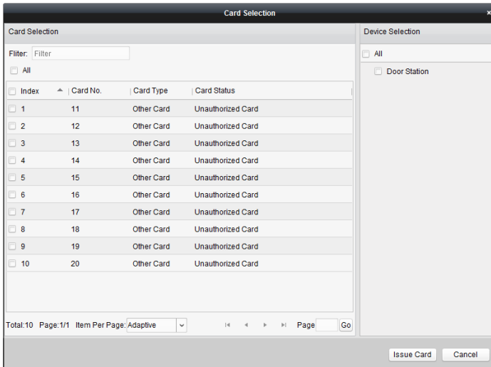
Рисунок 9-33 Выбор карт
