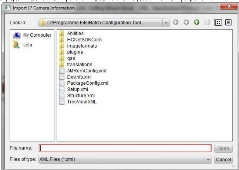
Рисунок 8-32 Импорт информации
