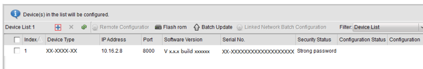
Рисунок 8-9 Кнопка добавления
