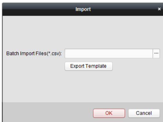
Рисунок 9-38 Импорт файлов
