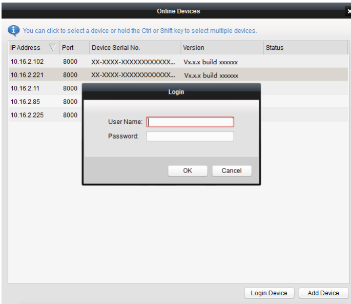
Рисунок 8-39 Окно авторизации
