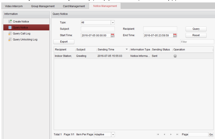
Рисунок 9-41 Меню уведомлений
