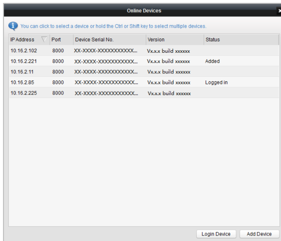
Рисунок 8-40 Устройства онлайн
