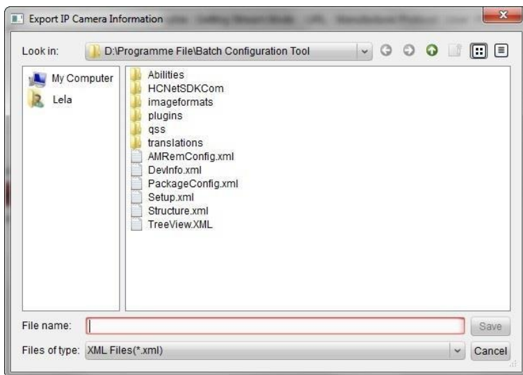
Рисунок 8-31 Экспорт информации
