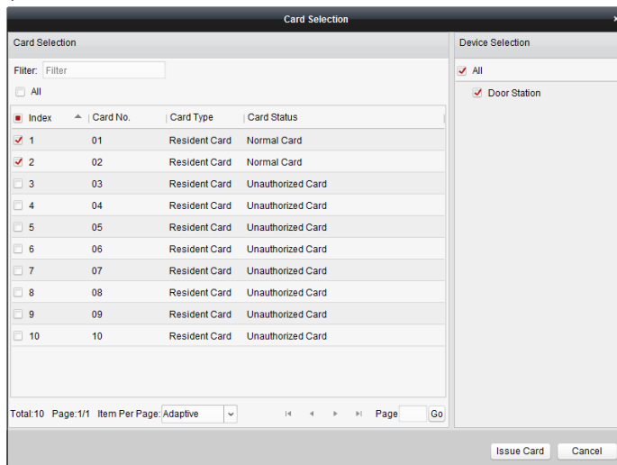
Рисунок 9-36 Выбор карт
