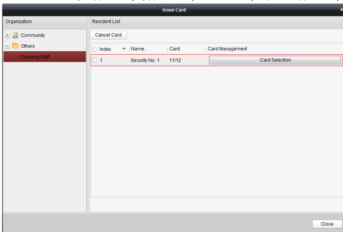
Рисунок 9-34 Выданные карты
