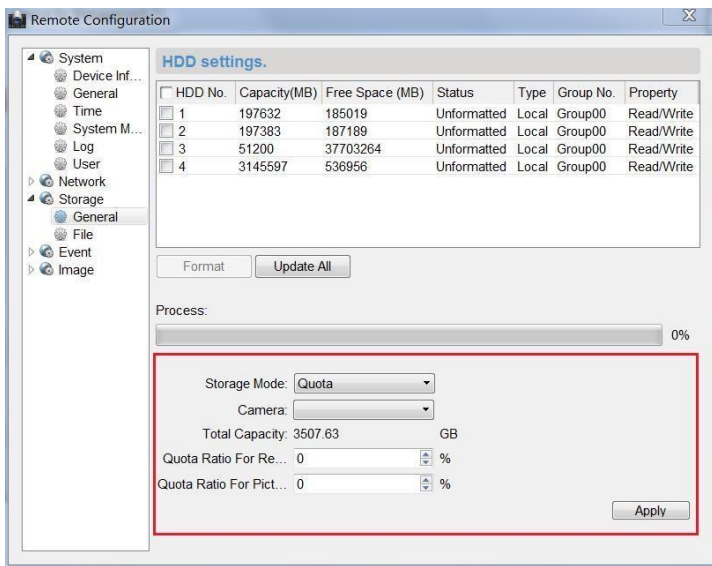
Рисунок 9-11 Настройка значения
