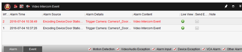
Рисунок 9-47 Аварийные события
