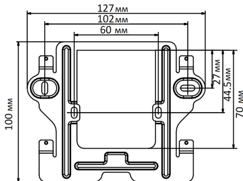
Рисунок 5-1 Монтажная пластина
