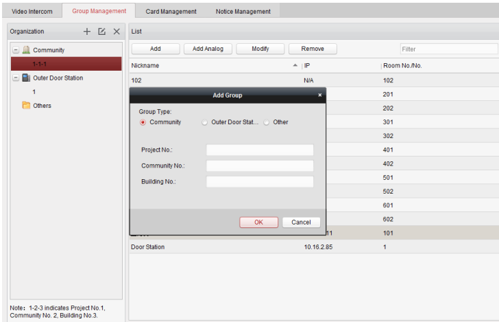
Рисунок 9-13 Добавление группы
