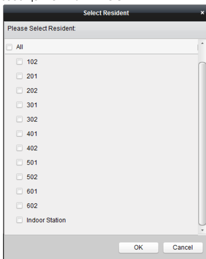
Рисунок 9-40 Выбор жильцов
