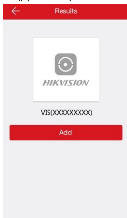
Рисунок 10-12 Результат поиска
