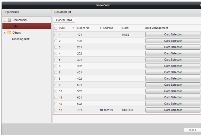
Рисунок 9-31 Выданные карты
