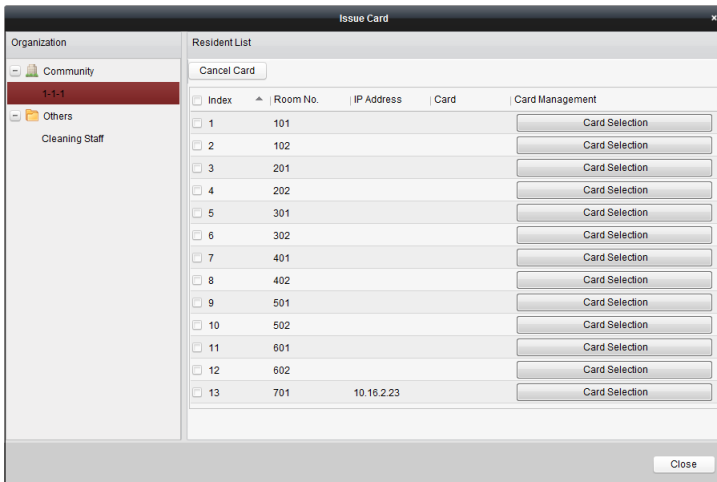
Рисунок 9-29 Выбор карт
