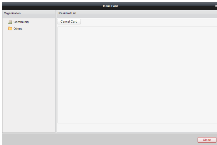
Рисунок 9-28 Выдача карт
