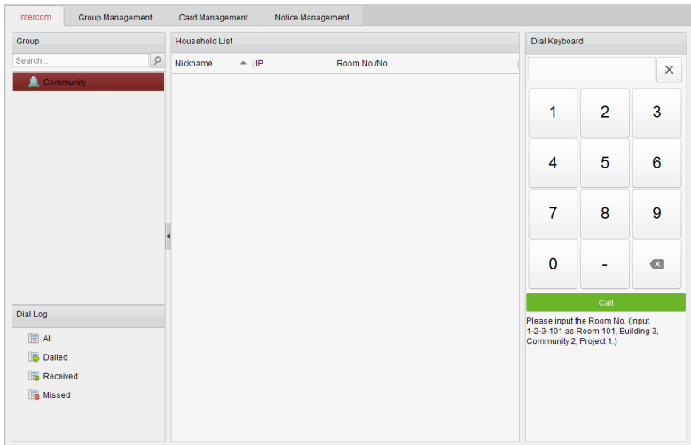
Рисунок 9-12 Меню домофона
