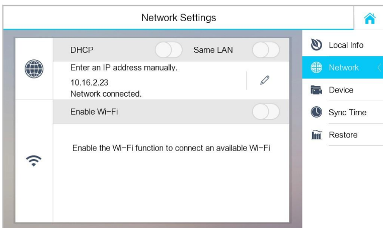
Рисунок 7-21 Интерфейс сети
