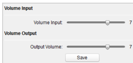
Рисунок 8-26 Конфигурация громкости
