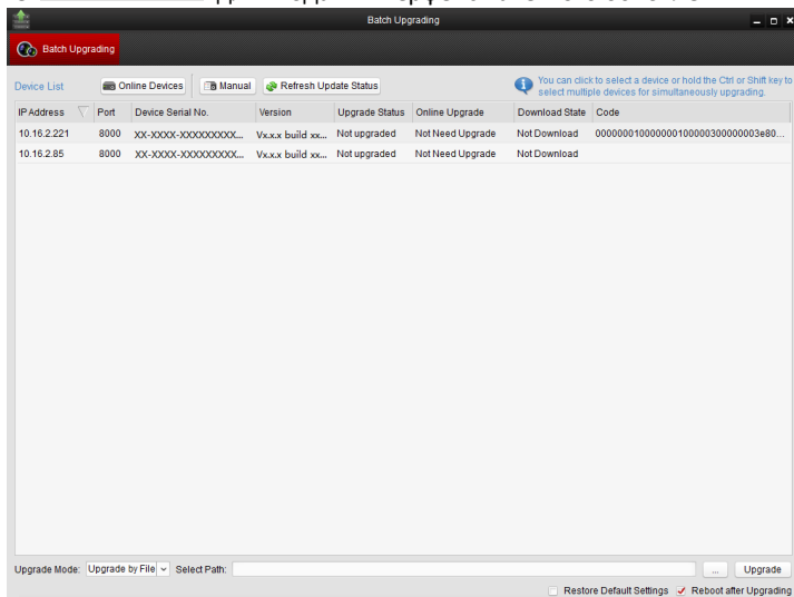
Рисунок 8-38 Пакетное обновление
