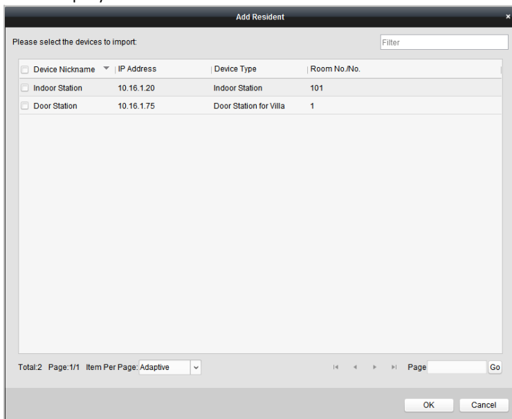
Рисунок 9-17 Добавление жильца
