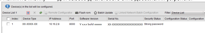
Рисунок 8-7 Кнопка добавления
