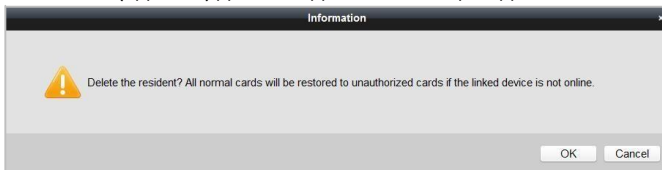
Рисунок 9-21 Информация
