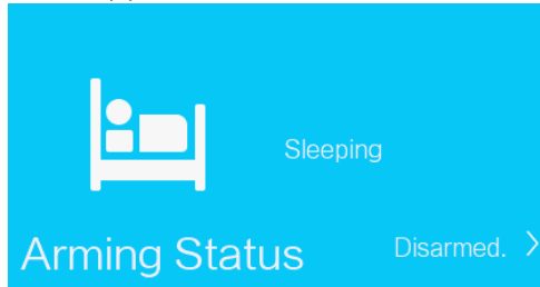
Рисунок 7-7 Режим «Сон»
