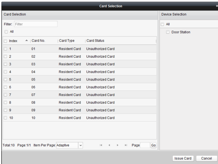
Рисунок 9-30 Выбор карт
