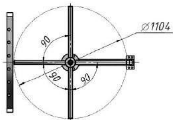
B-B (1 : 15)
