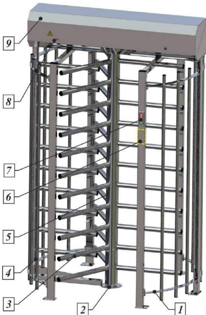
Рис. 2 – Конструкция и общий вид серии турникетов «Sesame» АЮИА.425
