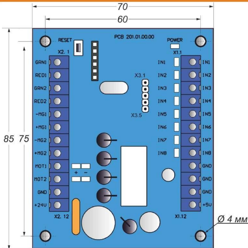
Рис.6 – Внешний вид контроллера PCB.201.01.00.00
