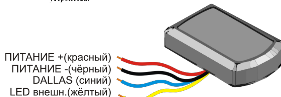
Рис.2. Схема подключение считывателя
