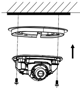
Рисунок 2-4 Установка камеры
