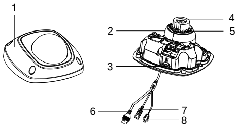
Рисунок 1-1 Внешний вид камеры I типа
