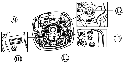
Рисунок 1-3 Внешний вид камеры II типа (2)
