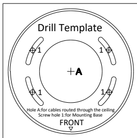
Рисунок 2-1 Шаблон крепления
