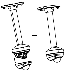
Рисунок 2-12 Установка крышки камеры
