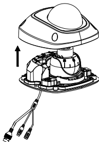
Рисунок 2-2 Демонтаж камеры
