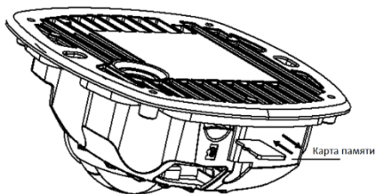
Рисунок 2-18 Установка microSD карты
