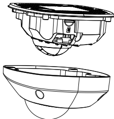
Рисунок 2-17 Удаление крышки камеры
