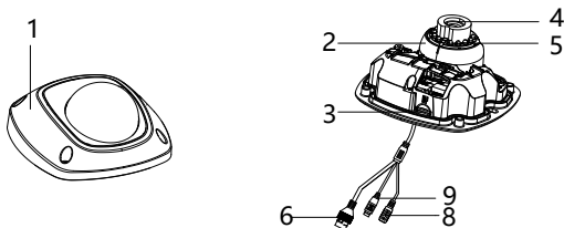
Рисунок 1-2 Внешний вид камеры II типа (1)
