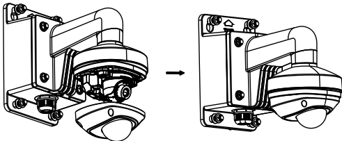
Рисунок 2-16 Установка крышки камеры
