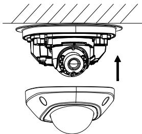
Рисунок 2-6 Установка крышки камеры
