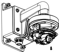
Рисунок 2-15 Установка камеры
