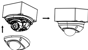
Рисунок 2-9 Установка крышки камеры
