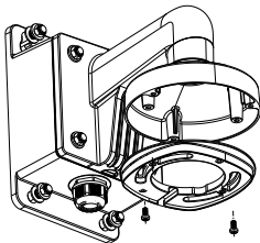
Рисунок 2-14 Установка монтажной платформы на кронштейн
