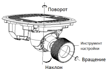
Рисунок 2-5 3-х осевая установка
