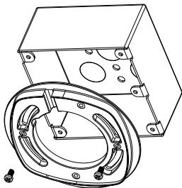
Рисунок 2-7 Установка монтажной платформы
