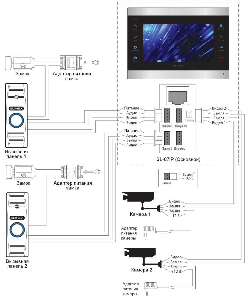
Схема 1. Подключение вызывных панелей и камер к домофону SL-07IP.
