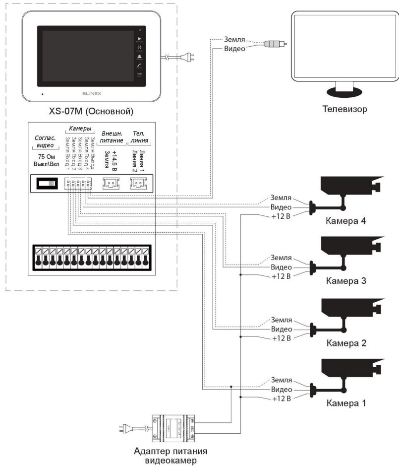
Схема 2. Подключение видеокамер и телевизора к домофону XS-07М
