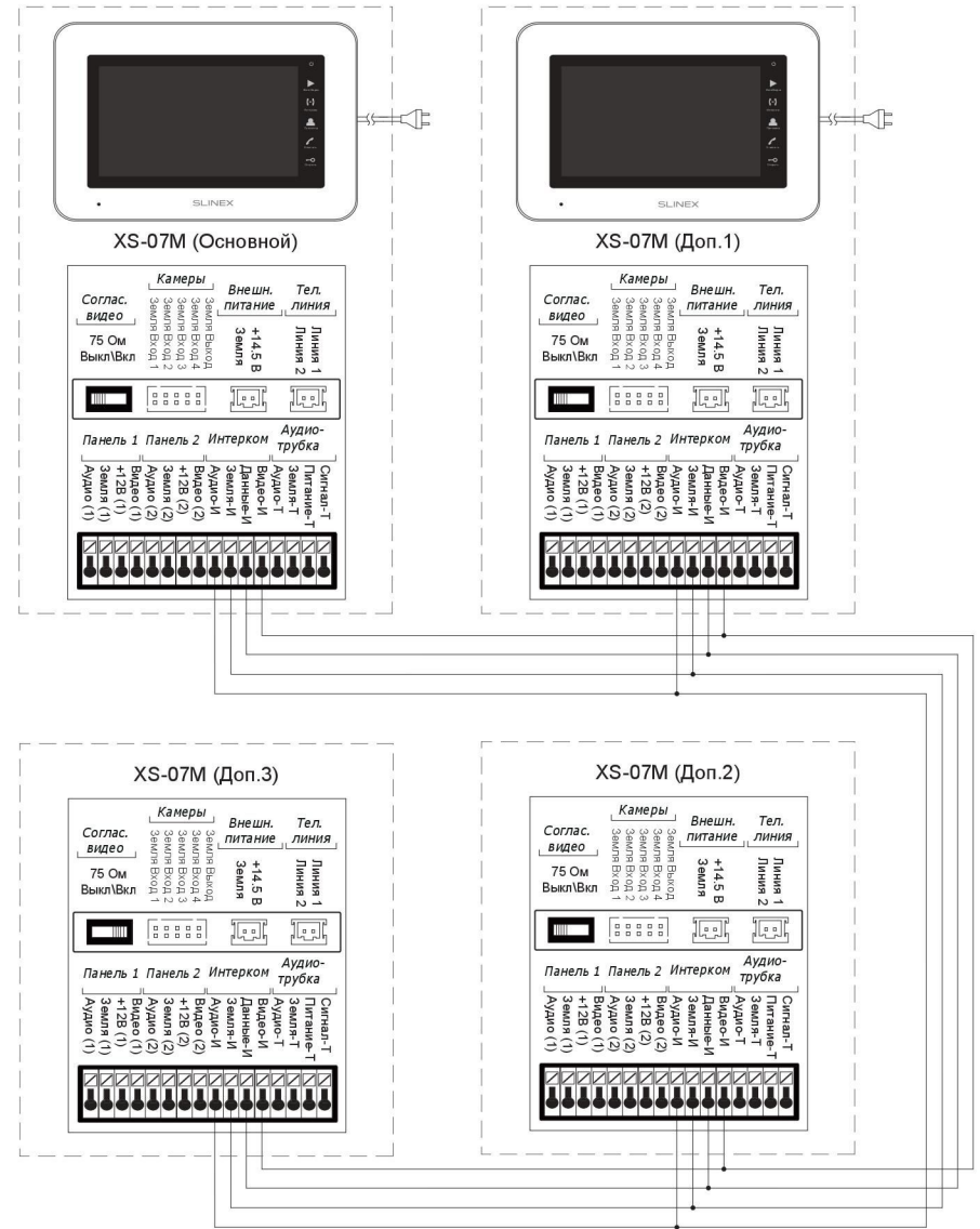
Схема 3. Подключение системы домофонов XS-07М в режиме CCTV1 – камеры могут быть подключены к любому монитору в системе. При этом просмотр камер возможен только на мониторе, к которому они подключены.
