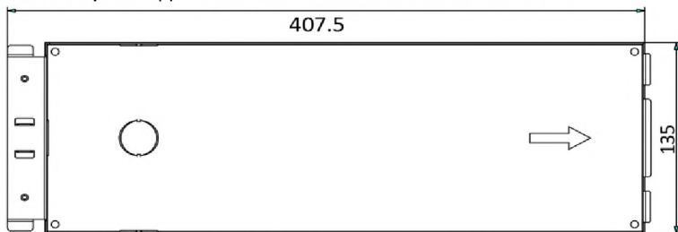
Рисунок 5-6 Вид спереди
