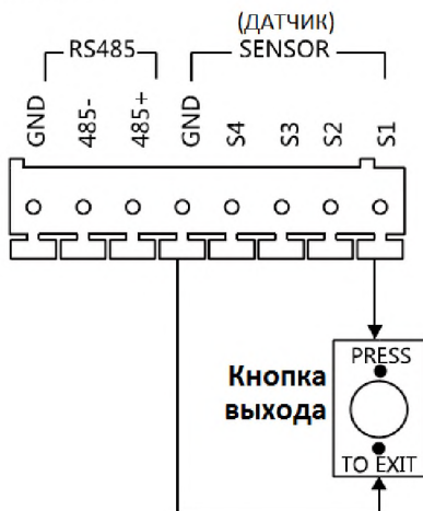
Рисунок 5-21 Подключение кнопки выхода для моделей DS-KD8102-V/DS-KD8002-VM (2)
