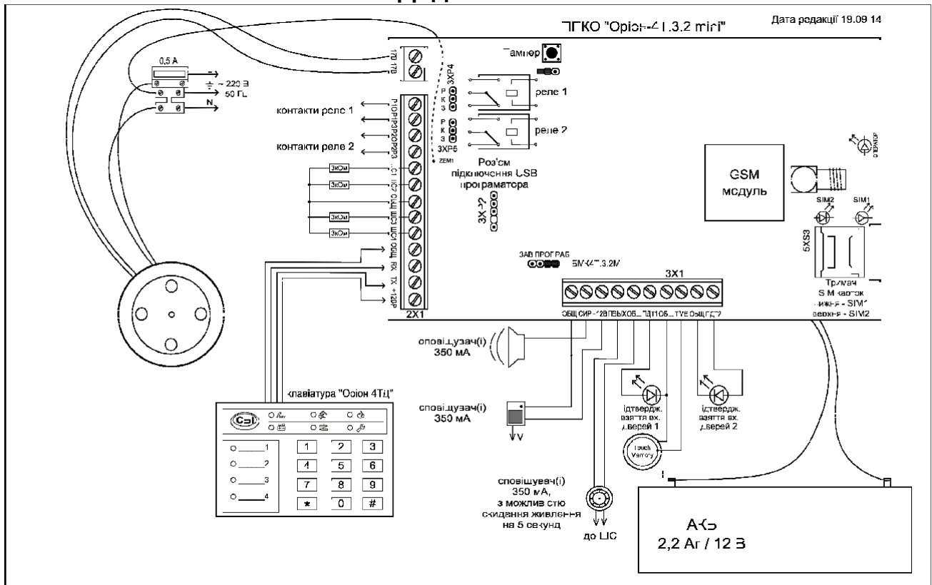
Рисунок А.1 - Схема електрична підключення ППКО «Оріон-4Т.3.2 mini»
